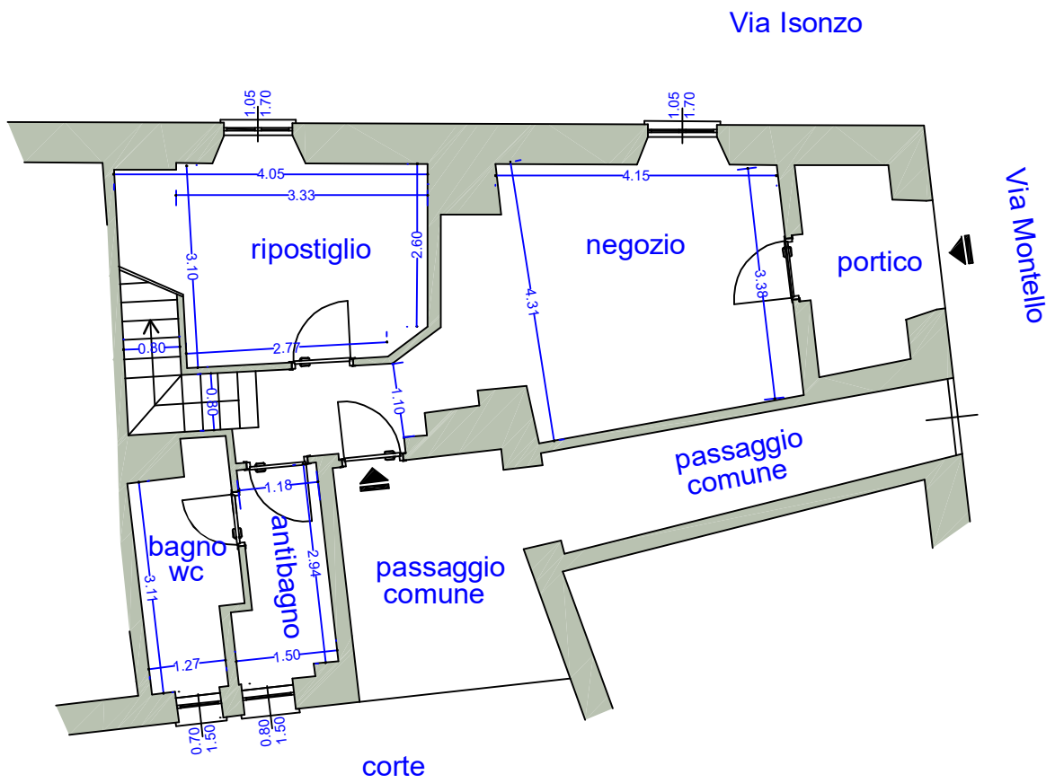
piano terra sc. 1:100
